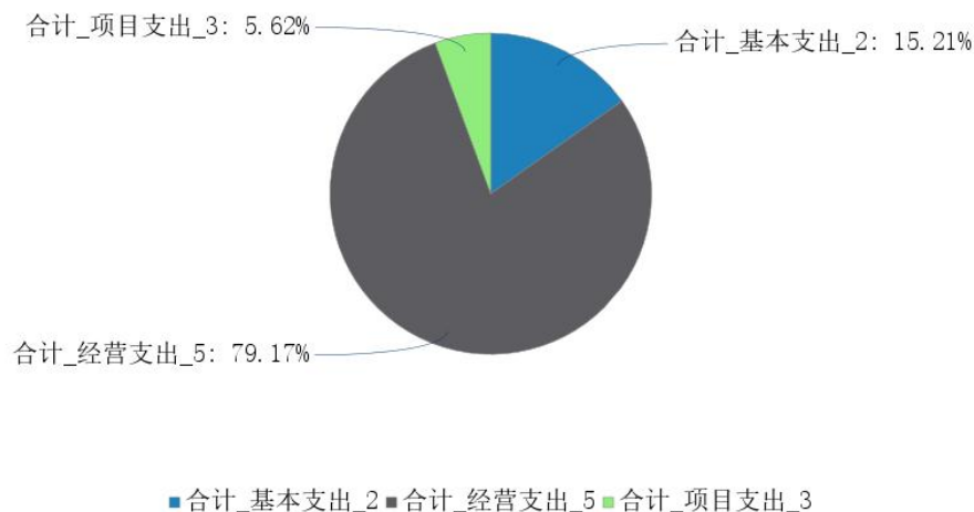
图2.支出决算图
